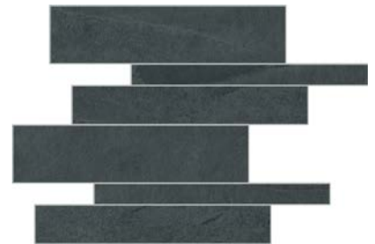
Linear Mosaic
